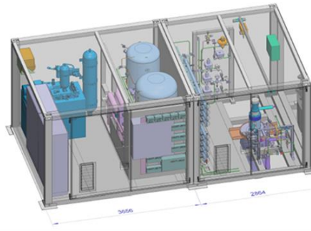
CP – Cryopump (LH2)
